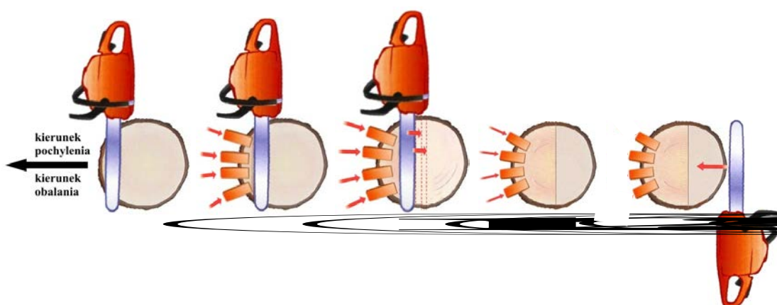
Rys.25 Technika ścinki i obalania drzewa silnie pochyłonego zgodnie z kierunkiem obalania z zastosowaniem metody „przez kliny” - średnica pnia mniejsza od użytecznej długości prowadnicy.
